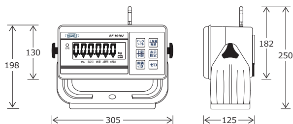
手元無線表示器 RF-1010J 外形寸法図 単位 mm
